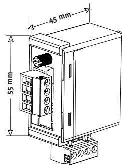
I/O module
