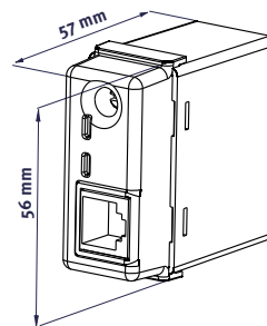
Ethernet module
